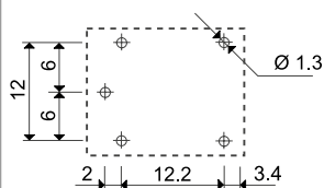
Csatlakozók nézetei
