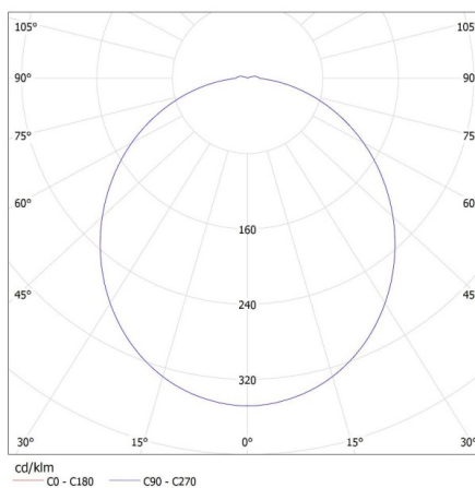
KANLUX S.A. (kat 32943) BENO 18W NW-L-GR / LDC (Polar)
