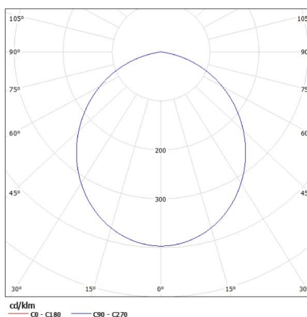
KANLUX S.A. (kat 23520) IMBER LED NW / Krzywa rozsyłu światła (biegunowo)
