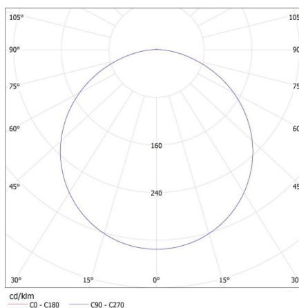
KANLUX S.A. (kat 26520) SANZO LED 15W-NW-SE / Krzywa rozsyłu światła (biegunowo)
