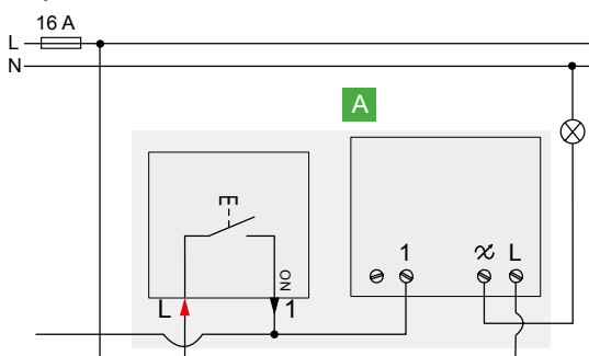
Egypólusú nyomó + Wiser fényerőszabályzó mikromodul (CCT5010-0002)
