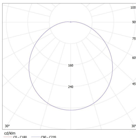
KANLUX S.A. (kat 19063) DABA N LED SMD DL-22W / Krzywa rozsyłu światła (biegunowo)
