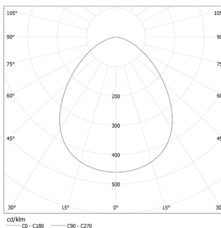
KANLUX S.A. (kat 25783) IVIAN LED 4,5W SN-NW / LDC (Polar)
